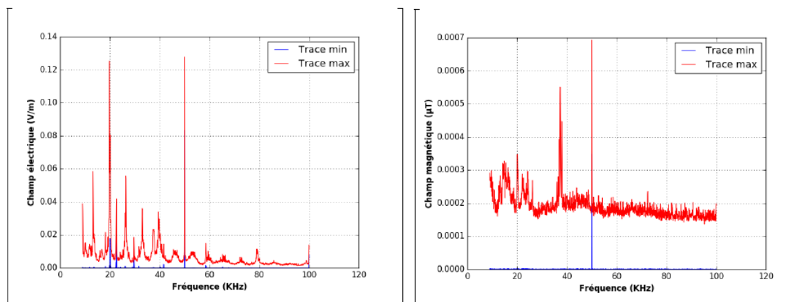
Figure 8 : illustration des niveaux de champs électrique à gauche et magnétique à droite en fonction de la fréquence dans le cas d'un compteur ne transmettant pas de CPL
