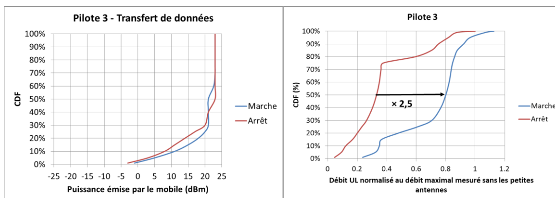
Figure 11 : distribution cumulative de la puissance émise par le mobile et du débit instantané enregistrés sur les parcours du pilote 3 avec les petites antennes en marche (courbes bleues) et éteintes (courbes rouges).
