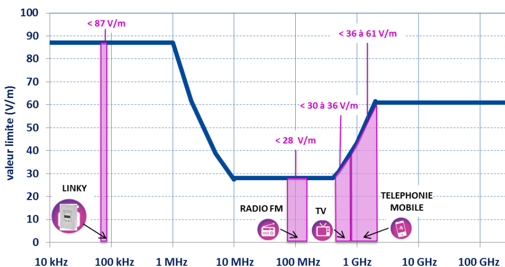
Figure 5 : valeurs limites réglementaires fixées en France par le décret du 3 mai 2002 n° 2002-775
