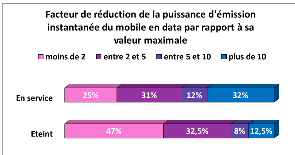
Figure 16: facteurs de réduction de la puissance instantanée d'émission du mobile lors de l'envoi de données par rapport à sa valeur maximale, obtenus sur les parcours dans les zones de 100 m autour des sites.
