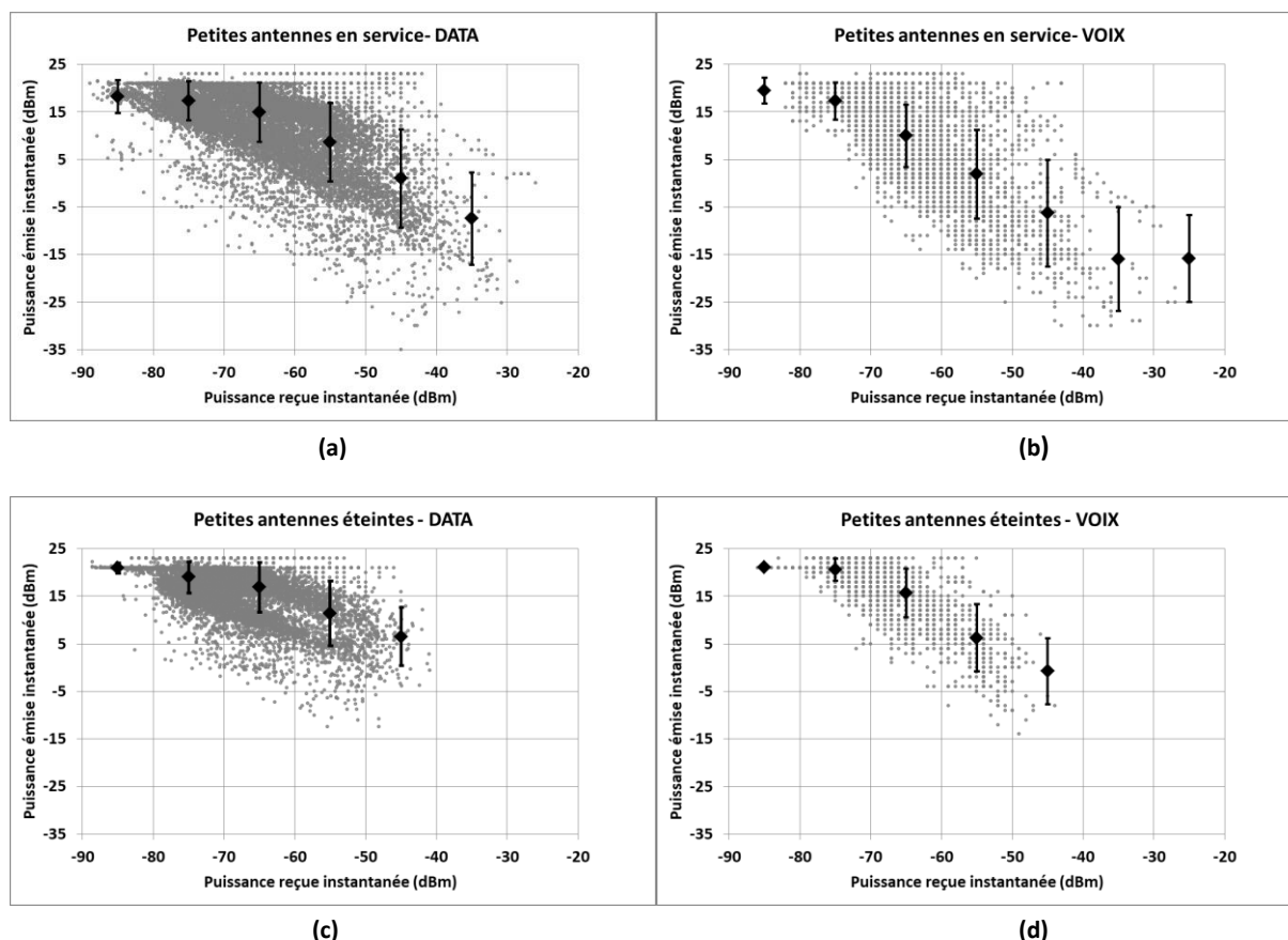
Figure 13 : lien entre la puissance émise instantanée par le mobile et la puissance instantanée reçue depuis le réseau par le mobile lors d'envoi de données lorsque les petites antennes sont en service (a) ou éteintes (c) et lors d'appels voix lorsque les petites antennes sont en service (b) ou éteintes (d). Les points gris sont l'ensemble des enregistrements, les losanges noirs sont les valeurs moyennes des puissances émises obtenues sur des intervalles de 10 dBm de puissances reçues et les traits noirs correspondent à l'intervalle d'un écart type qui matérialise la dispersion des valeurs de puissances émises autour de la valeur moyenne.
