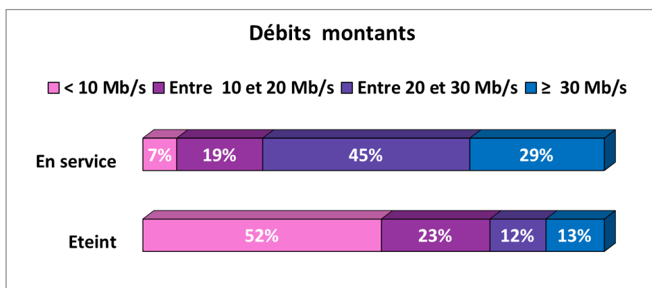
Figure 17 : débits montants mesurés lors de l'envoi de données obtenus sur les parcours dans les zones de 100 m autour des sites.
