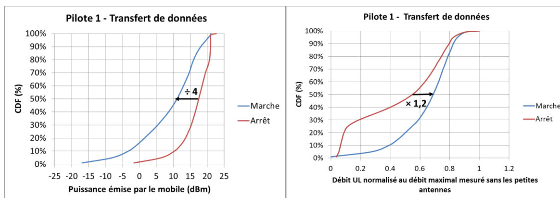
Figure 9 : distribution cumulative 5 de la puissance émise par le mobile et du débit instantané enregistrés sur les parcours du pilote 1 avec les petites antennes en marche (courbes bleues) et éteintes (courbes rouge).
