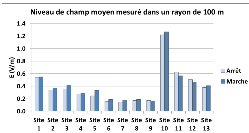
Figure 6 : niveau d'exposition moyen mesuré dans des zones de 100 mètres autour des sites quand les petites antennes sont arrêtées ou en marche
