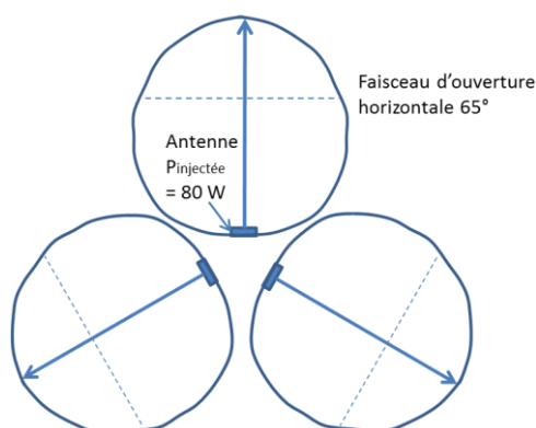
Figure 2 : vue de dessus d'un site comportant trois antennes macros
