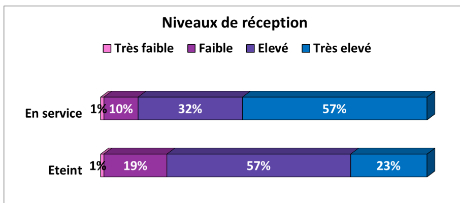
Figure 14 : niveaux de réception du réseau lorsque les petites antennes sont en marche ou arrêtées, obtenus sur les parcours dans les zones de 100 m autour des sites.
