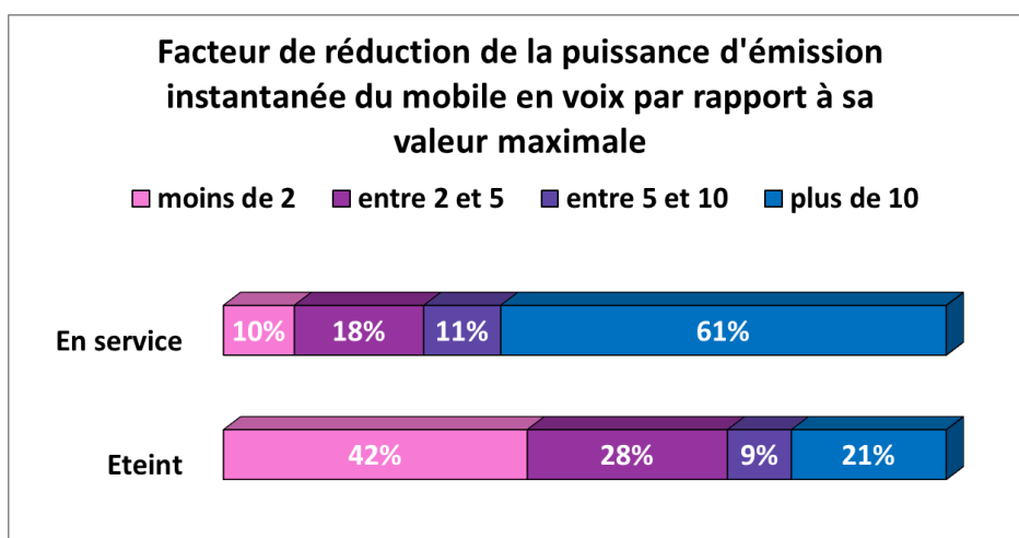
Figure 15 : facteurs de réduction de la puissance instantanée d'émission du mobile lors des communications voix par rapport à sa valeur maximale, obtenus sur les parcours dans les zones de 100 m autour des sites.
