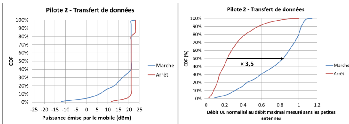
Figure 10 : distribution cumulative de la puissance émise par le mobile et du débit instantané enregistrés sur les parcours du pilote 2 avec les petites antennes en marche (courbes bleues) et éteintes (courbes rouges).
