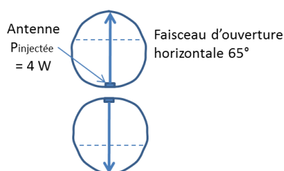
Figure 3 : vue de dessus d'un site micro contenant deux antennes micros
