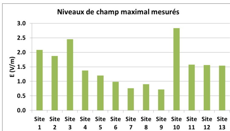
Figure 7 : niveaux maximaux mesurés à proximité des sites lorsque les petites antennes sont en marche
