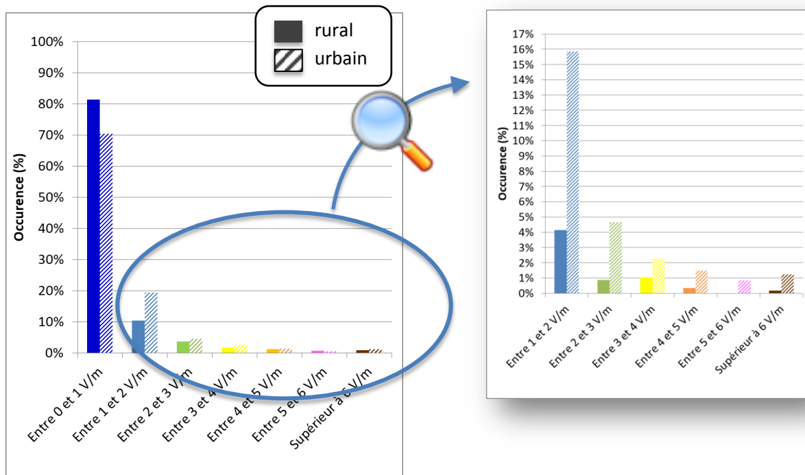
Figure 8 : comparaison des distributions des niveaux de champ électrique mesuré en milieu rural (barres pleines) et en milieu urbain (barres hachurées) et zoom sur les distributions au-delà de 1 V/m
